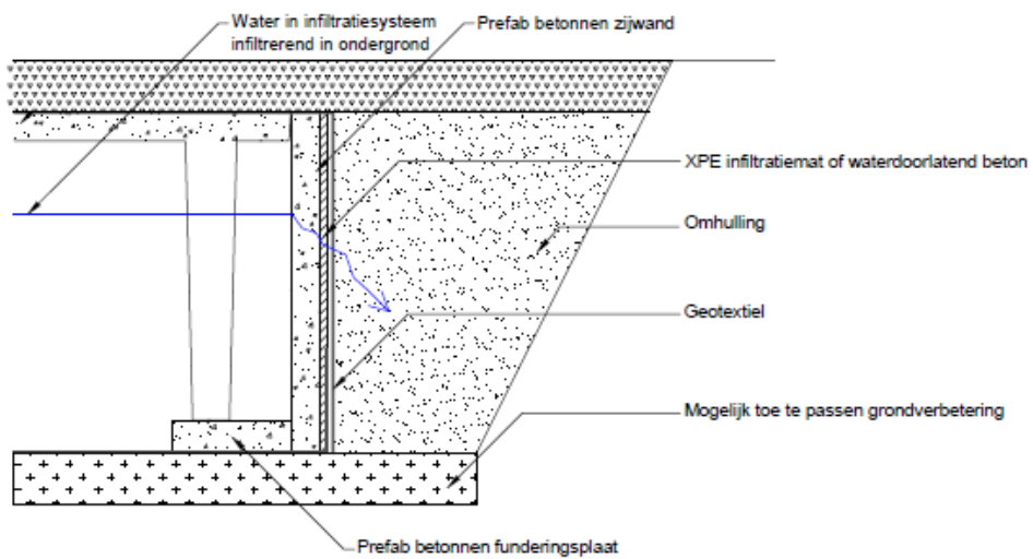
Doorsnede ter plaatse van zijwand incl. benoeming onderdelen
