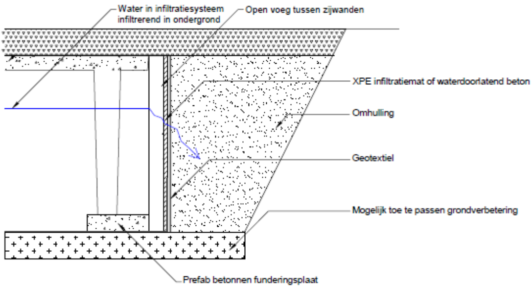
Doorsnede ter plaatse van voeg incl. benoeming onderdelen
