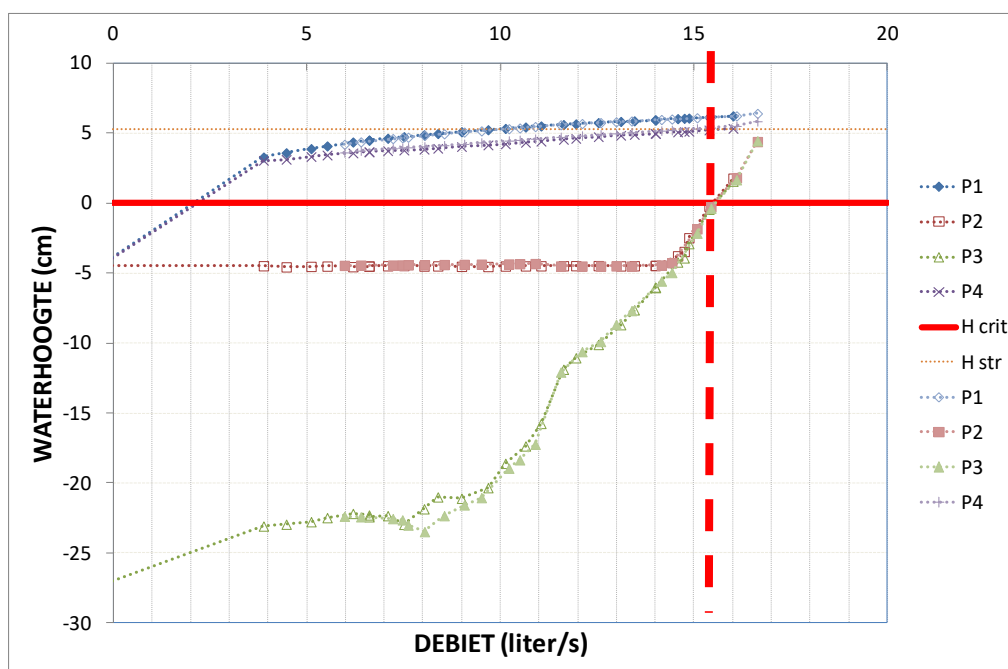
Figuur 2. De relatie tussen debiet en waterniveau (uitgemiddeld per stap) kan men beschouwen als de karakteristiek van de kolk. Waar de karakteristiek de (referentie)hoogte van de regengoot snijdt ( H = 0 cm) kan men de overeenkomstig debiet als de maximale doorvoercapaciteit van de kolk definiëren.
